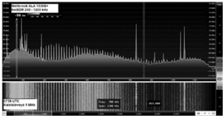
Wellbrook ALA1530S+ antennin signaalitasot keskiaaltoalueen alapäässä (200–1200 kHz, päiväkelit). Pohjataso esim. 270 kHz taajuudella on noin -97 dBm.
