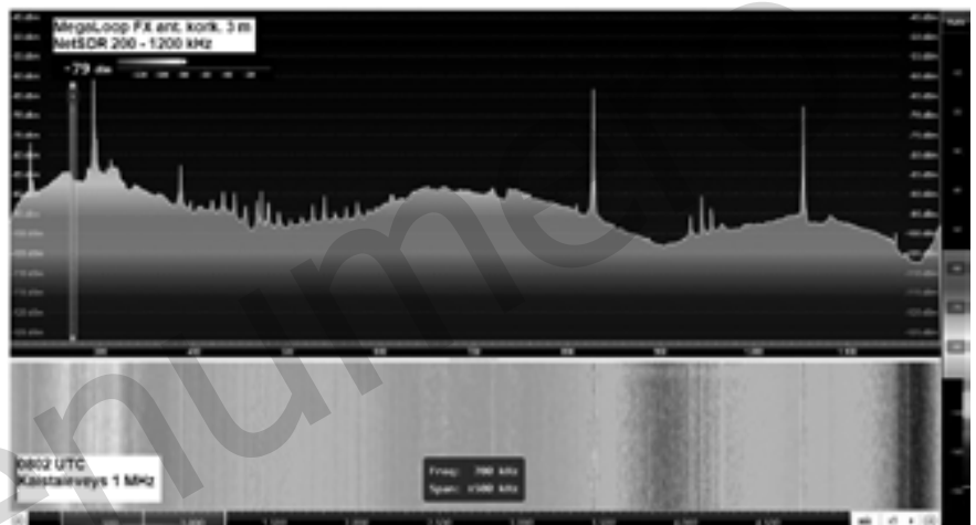
MegaLoop FX antennin signaalitasot keskiaaltoalueen alapäässä (200–1200 kHz, päiväkelit). Pohjataso esim. 270 kHz taajuudella on noin -87 dBm. Antennissa korostuvat myös 700 kHz ja 1050 kHz:n kohinamaksimit.
