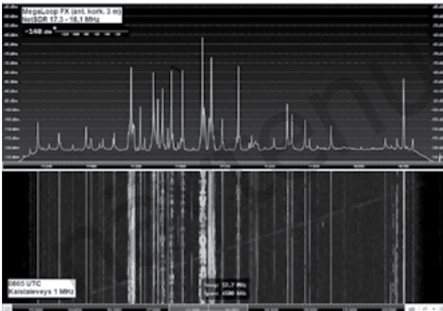
MegaLoop FX antennin signaalitasot 17,5 MHz BC-alueella (NetSDR/9 dB Clifton Labs -vahvistin/SpectraVue). Syyskuun päiväkelit, antennin sijoituskorkeus 3 metriä. Pohjataso on noin -122 dBm, signaalien huiput max. -62 dBm.
