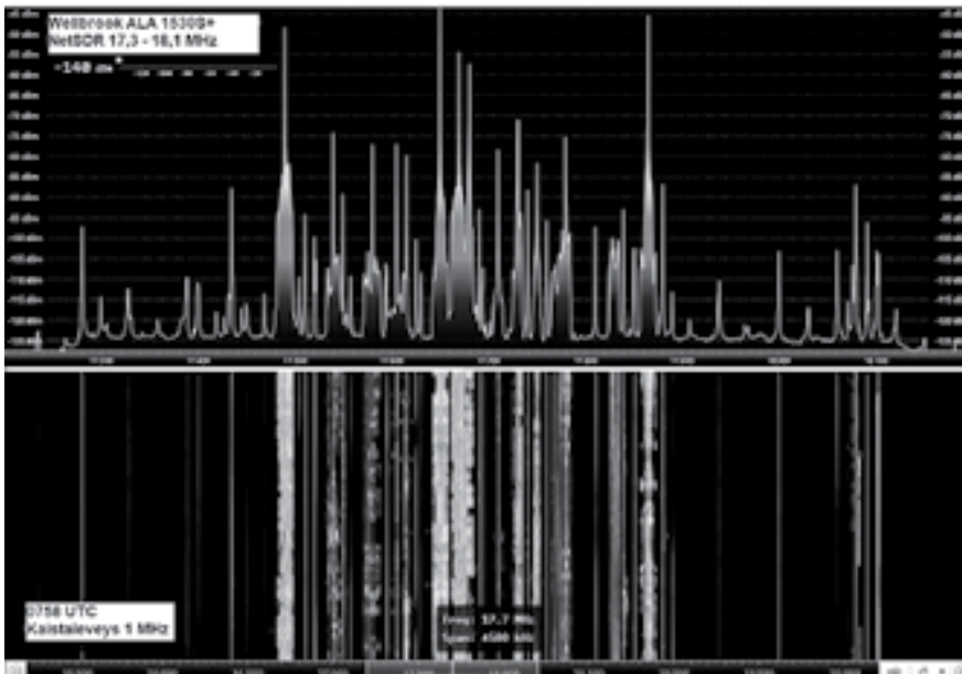
Wellbrook ALA 1530S+ antennin signaalitasot 17,5 MHz BC-alueella (NetSDR/9 dB Clifton Labs -vahvistin/SpectraVue). Syyskuun päiväkelit, antennin sijoituskorkeus 4 metriä. Pohjataso on noin -124 ... -125 dBm, signaalien huiput max. -43 ... -45 dBm.
